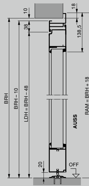
Zijdeur met aluminium hoekkozijn Buitenaanslag
