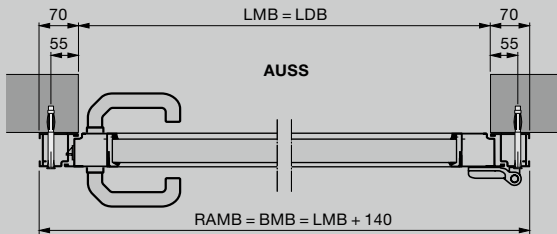
Zijdeur met aluminium blokkozijn Inbouw achter de opening
