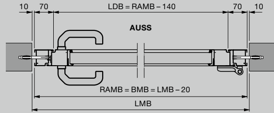
Zijdeur met aluminium blokkozijn Inbouw in de opening
