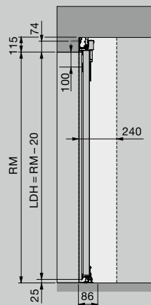
Wandmontage als schuifdeur
