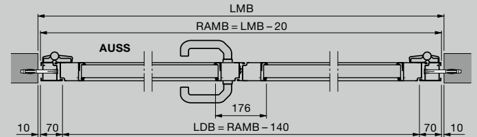
2-vleugelige zijdeur met aluminium blokkozijn Inbouw in de opening
