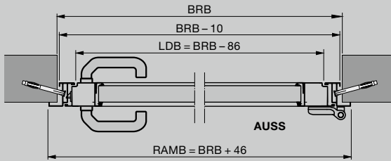
Zijdeur met hoekkozijn Inbouw voor de opening
